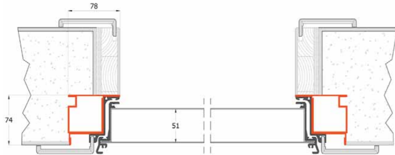
Soluzione 2 - Portone blindato a filo lato interno con mostrina, con imbotte in legno e mostrina lato esterno Solution 2 - Interior side security door with trim, with wood door jamb and exterior side trim
