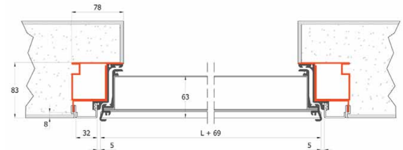
Soluzione 6 - Tipologia di installazione con telaio filomuro. Per le altre modalità segue la modalità generale delle varianti precedenti Solution 6 - Filomuro frame installation typology. Adopt the general procedure of the previous variants for the other procedures
