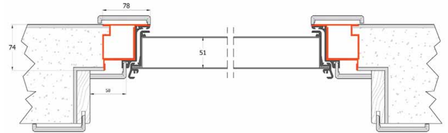
Soluzione 4 - Portone blindato a filo lato esterno con mostrina e imbotte lato interno e mostrina lato esterno Solution 4 - Exterior side security door with trim and door jamb side and exterior side
