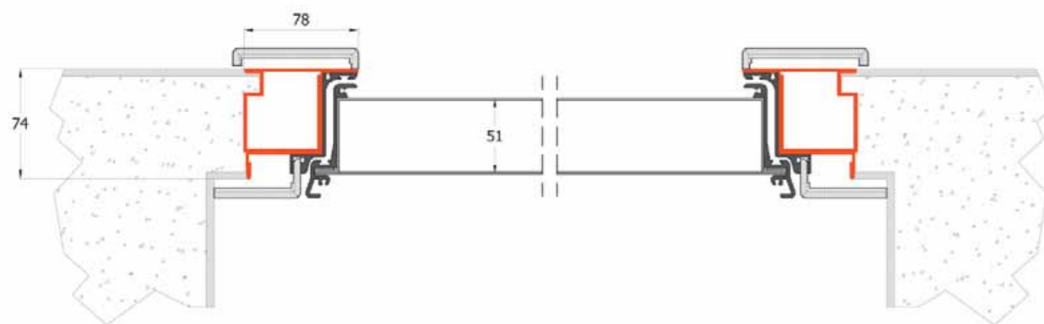
Soluzione 3 - Portone blindato a filo lato esterno con mostrina lato interno e lato esterno Solution 3 - Exterior side security door with trim interior side and exterior side
