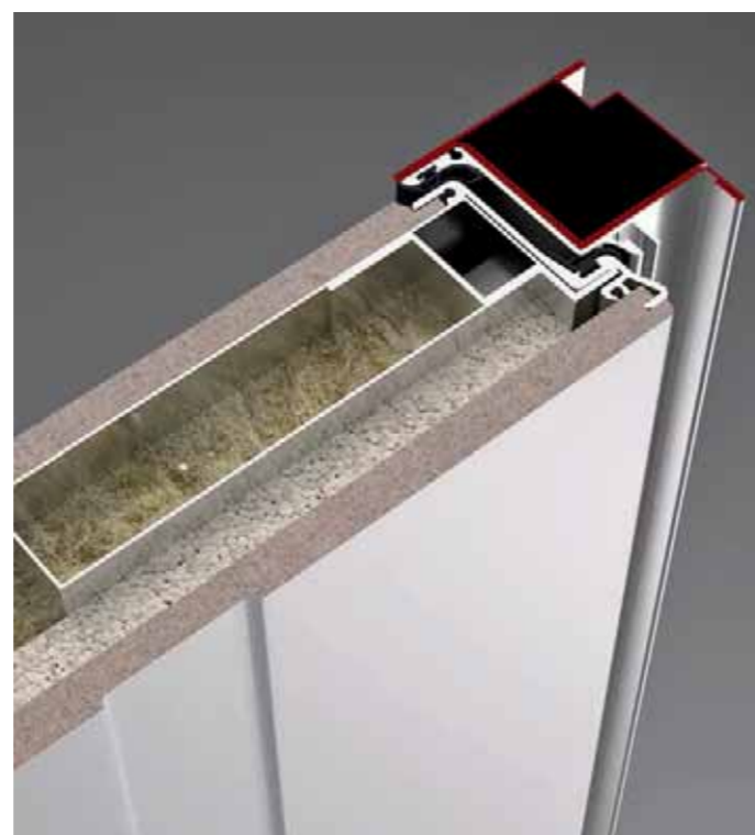
Pannello anta con spessore 14 mm, laccato o impiallacciato legno 14 mm thick lacquered or veneered wood door panel
