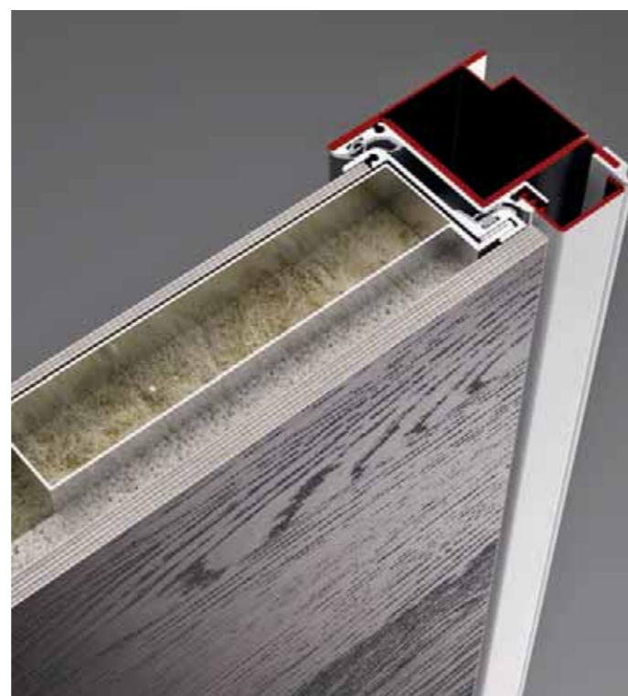
Pannello anta con spessore 9,5 mm tipologia Filomuro, laccato o impiallacciato legno 9.5 mm thick lacquered or veneered wood Filomuro door panel
