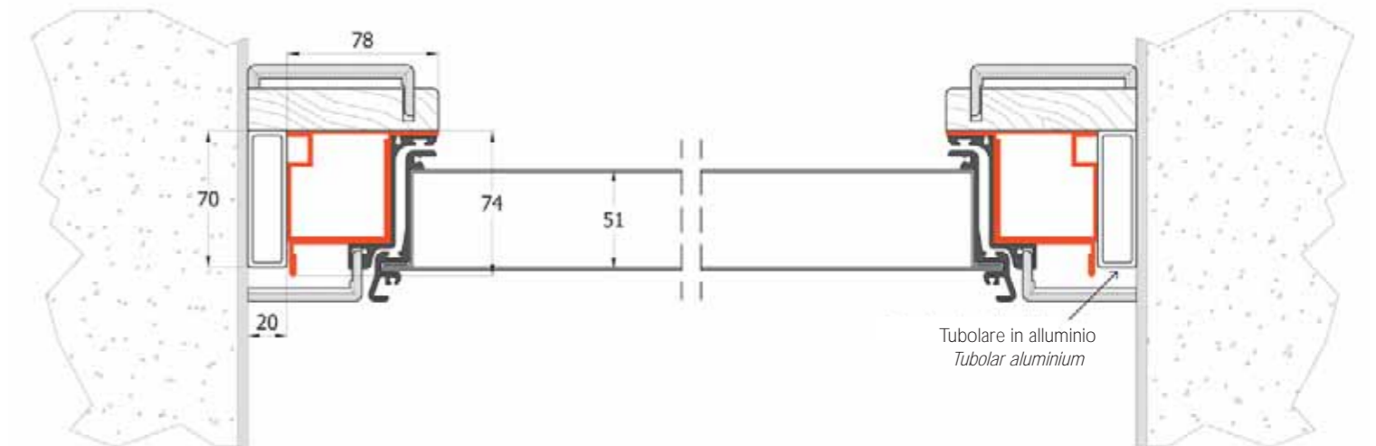
Soluzione 5 - Portone blindato montato a centro muro con profilo di compensazione Solution 5 - Security door mounted in the wall centre with off-setting profile
