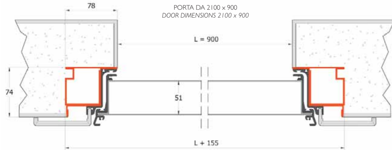
Soluzione 1 - Portone blindato a filo lato interno con mostrina Solution 1 - Interior side security door with trim
